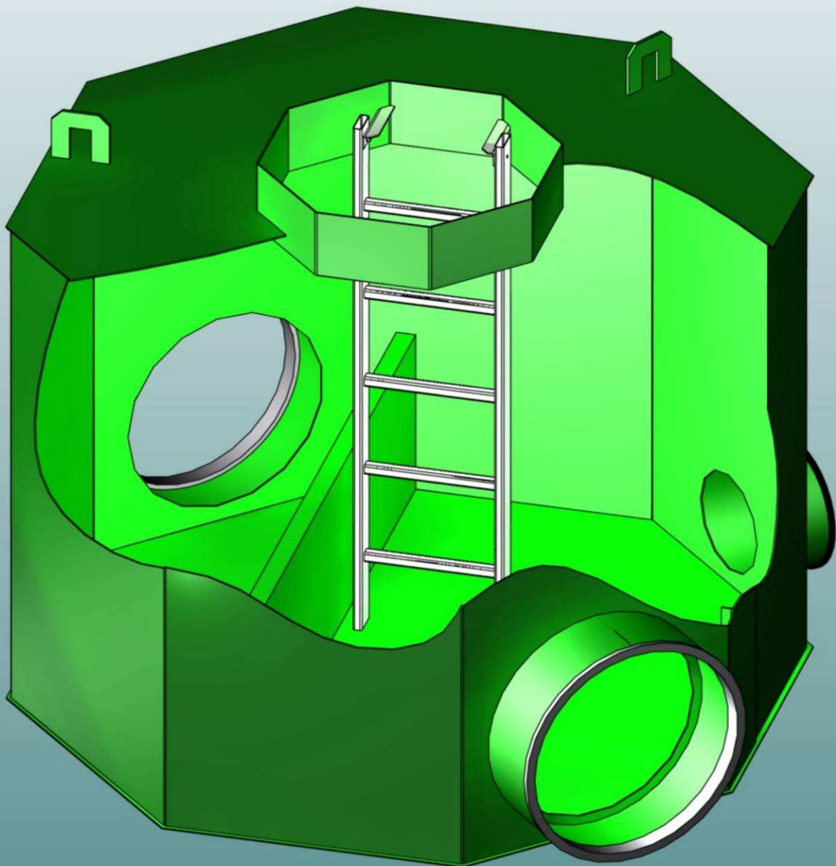
DEVERSOIR D'ORAGE type DV.0
